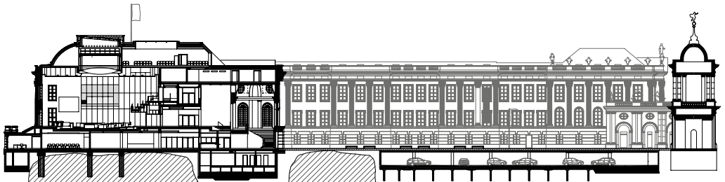
The Landtag building from the east in cross section (© Ministerium der Finanzen und für Europa des Landes Brandenburg)
